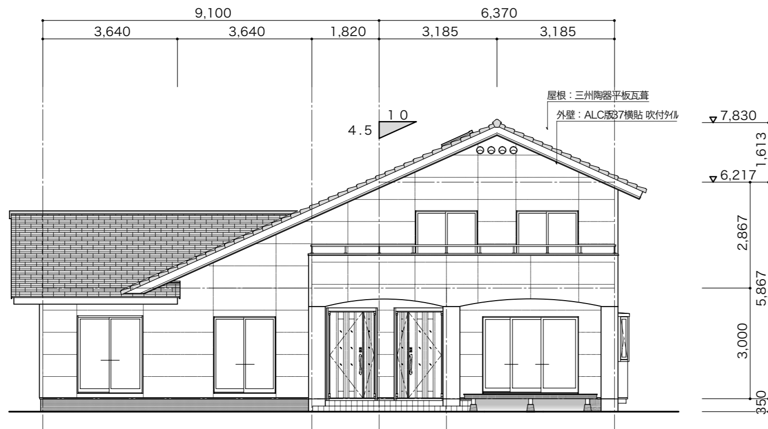
南立面図 S = 1 / 100
